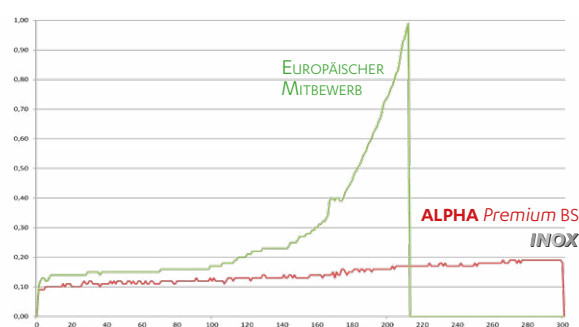
Verschleißtest: Alpha Premium INOX gegen rostfreie Qualitätskette europäischer Fertigung
